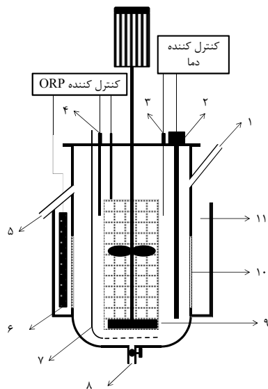
شکل (۲) تصویر شماتیک رآکتور مورد استفاده برای بیولیچینگ الکتروشیمیایی: (۱) ورودی خوراک، (۲) المنت حرارتی، (۳) سنسور دما، (۴) الکترود ORP، (۵) سرریز محصول، (۶) الکترود آند، (۷) لوله هوادهی، (۸) شیر تخلیه، (۹) الکترود کاتد، (۱۰) غشاء تبادل یون، (۱۱) محفظه آندی
