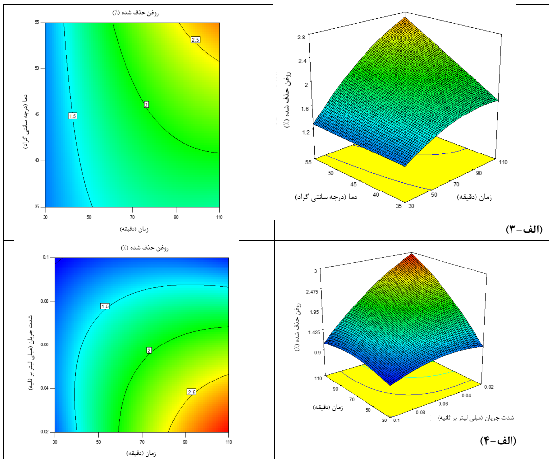
شکل (۳) نمودار سه بعدی و کانتور تأثیر متغیرهای مستقل بر بازیافت خاک به روش فوق‌بحرانی؛ الف-۱: فشار و دما، الف-۲: زمان و فشار، الف-۳: زمان و دما، الف-۴: زمان و شدت جریان.
