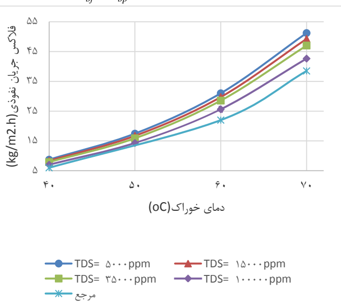
شکل ۴- تغییرات محصول تقطیر غشایی با دمای خوراک و شوری
