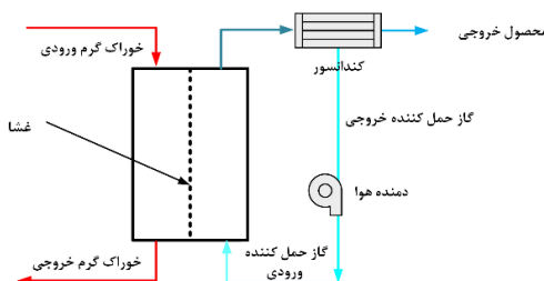
ج. تقطیر غشایی با گاز حمل کننده
