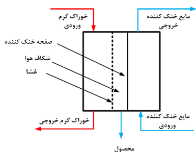
ب. تقطیر غشایی با لایه هوا
