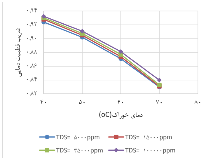
شکل ۵- تغییرات ضریب قطبیت دمایی با شوری خوراک
